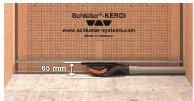
Niedrige Einbauhöhe: 65 mm
